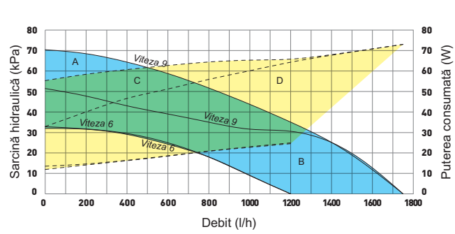
Grafic debit/sarcină hidraulică VICTRIX TERA V2 38 EU/ VICTRIX TERA V2 35 PLUS EU
