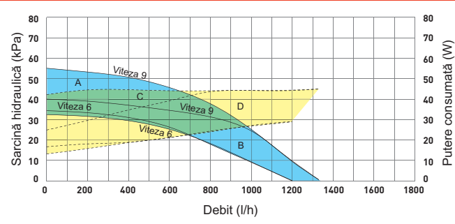
Grafic debit/sarcină hidraulică VICTRIX TERA V2 28 EU/VICTRIX TERA V2 24 PLUS EU
