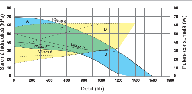
Grafic debit/sarcină hidraulică VICTRIX TERA V2 32 EU
